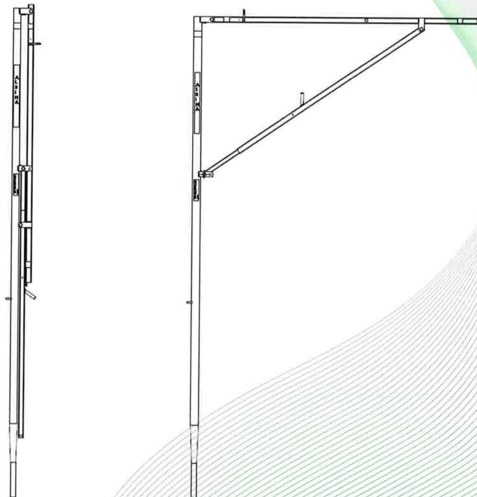
Ilustración 1: Dispositivo de anclaje, tipo: Alsipercha
