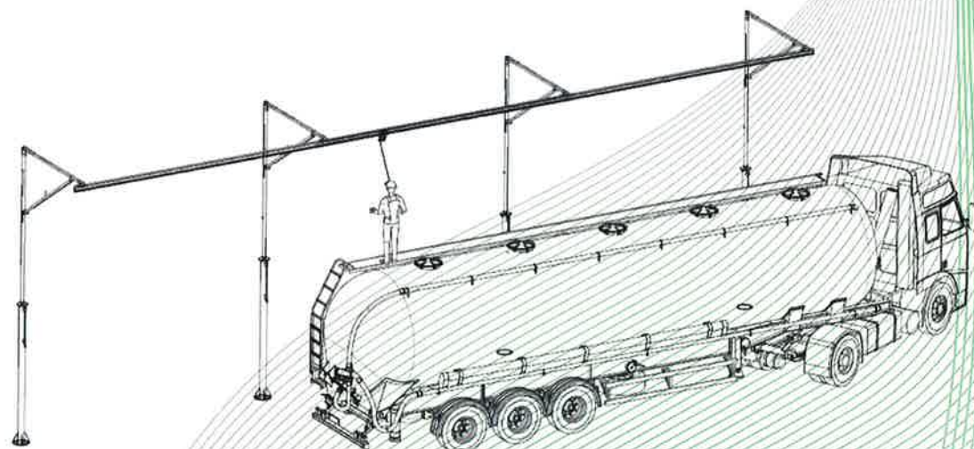
Ilustración 7: Dispositivo de anclaje del tipo D (tipo: Horizontal Safeaccess y NAV2 trolley / fabricante: FALLPROTEC SA) con anclajes, tipo: AluPercha y Post for reduced spaces
