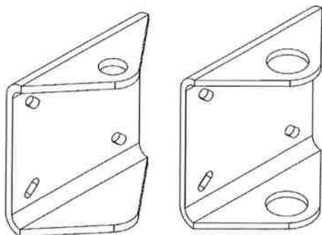
Ilustración 5: Anclaje, tipo: Wall brackets
